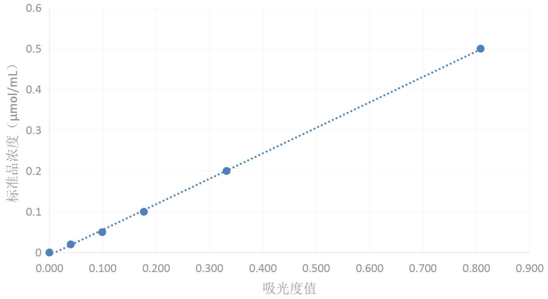
土壤碱性蛋白酶标准曲线
